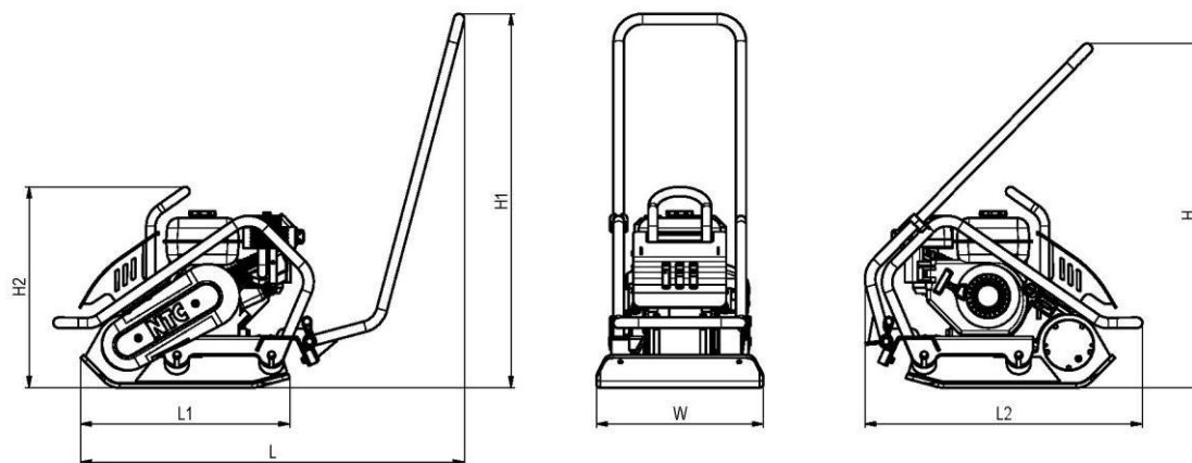
Obr. Základní popis stroje – varianta bez kropíciho zařízení
